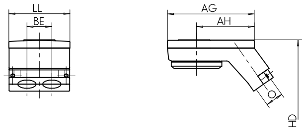
Standanschlusskasten für Kabelvergussstutzen
