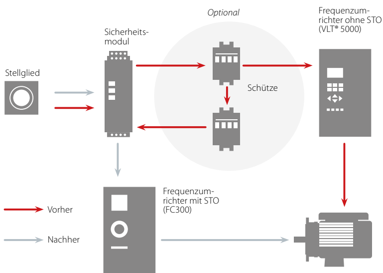
Zwei Schütze können bei der Sicherheitsinstallation dank der Sicherheitsfunktionalität des VLT® AutomationDrive wegfallen.
