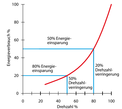
50 % Energieeinsparungen, wenn die Lüfterdrehzahl von 100 % auf 80 % reduziert wird.
